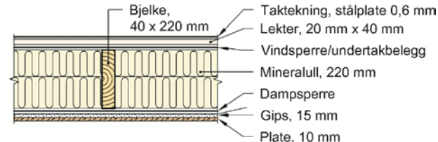
Fig 4 Prinsipiell oppbygging av takkonstruksjonen over modulen. Bjelker har avstand c/c 600 mm.
