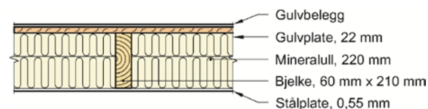
Fig. 3 Prinsipiell oppbygging av golv i modulene. Trebjelker har avstand c/c 625 mm.
